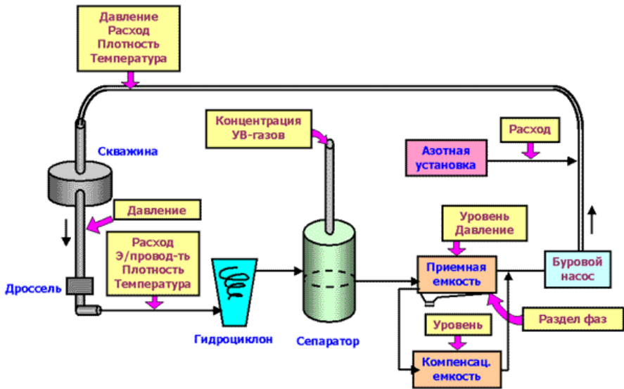
Рисунок 2. Схема размещения датчиков в закрытой циркуляционной системе для вскрытия пластов на депрессии.
