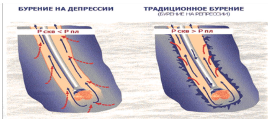
Рисунок 1. Взаимодействие в системе «скважина – пласт» при бурении на депрессии и репрессии.
